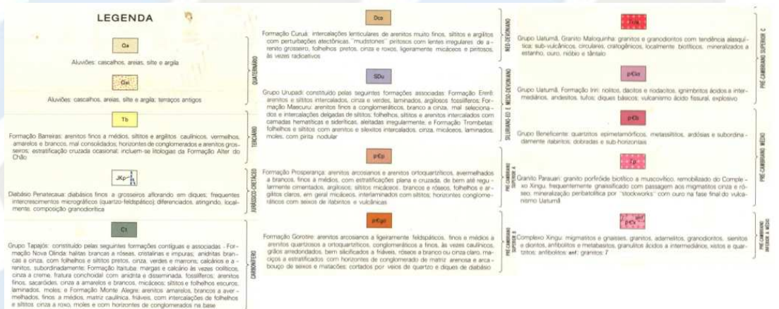
Figura 4 - Localização – Mapa Geológico (Folha SB-21-X-A Itaituba)
